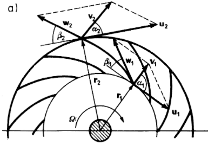
Wirnik promieniowy
