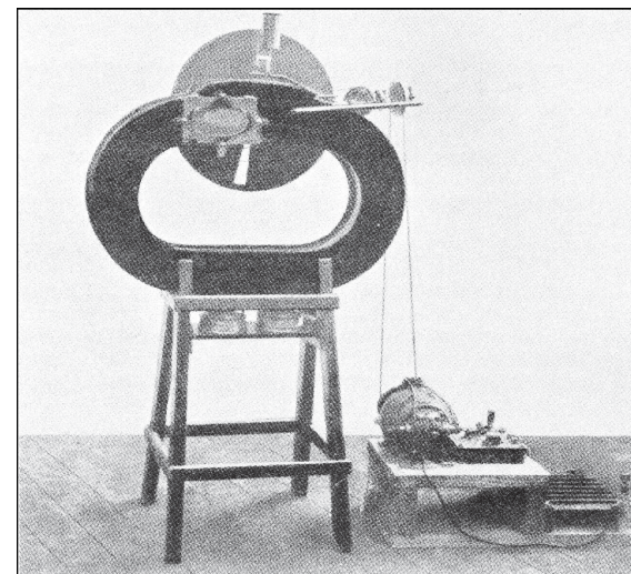
Pierwszy tunel kawitacyjny zbudowany przez Parsonsa 1895
